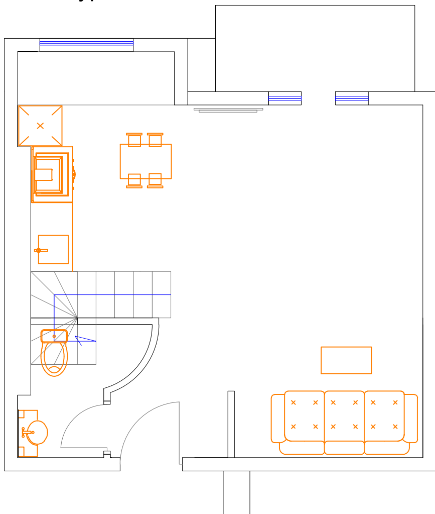
план 1 уровня
